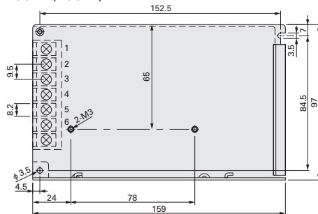
ESP10-150-*(150W)
