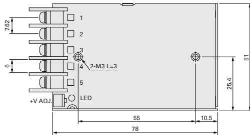
ESP10-50-*(50W)
