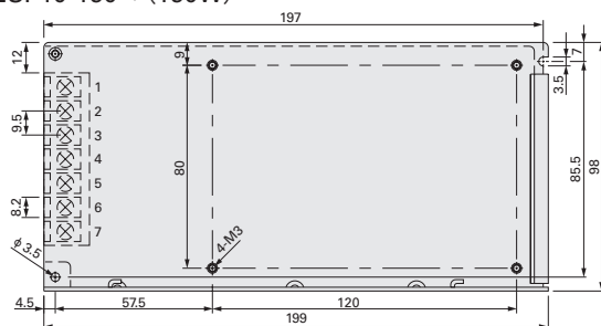
ESP10-150-*(150W)
