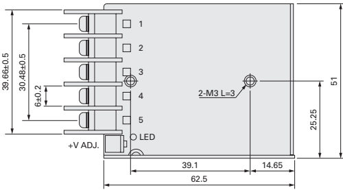
ESP10-25-*(25W)
