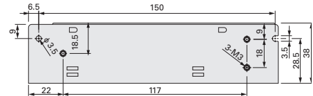
端子台脚位定义
