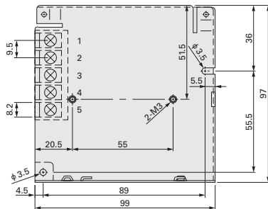
ESP10-100-*(100W)
